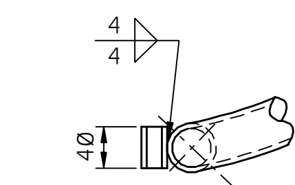
J SECTION - SCALE 1 : 5
