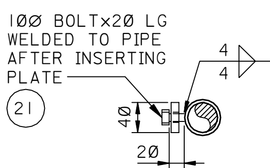
M SECTION - SCALE 1 : 5
