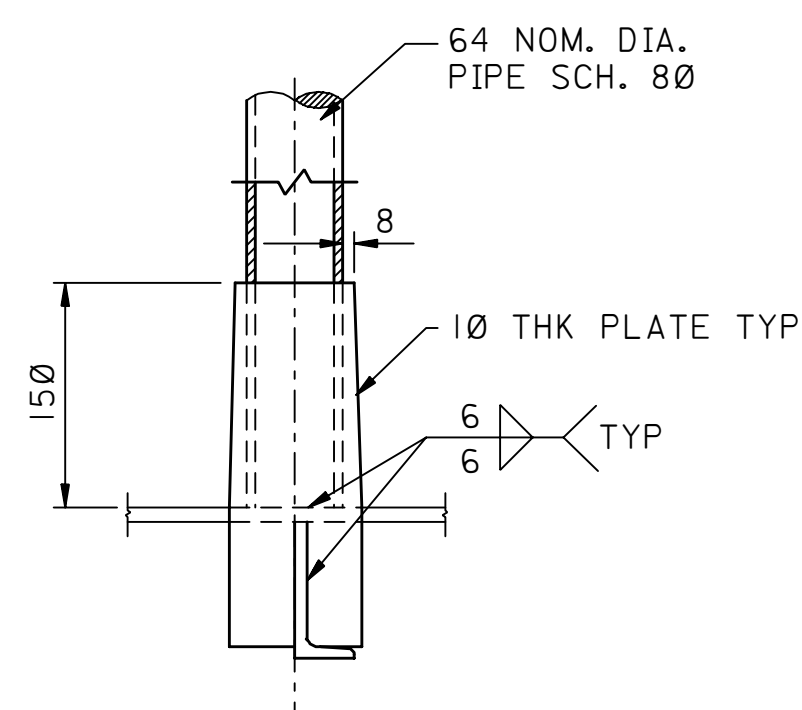
G SECTION SCALE 1 : 5
