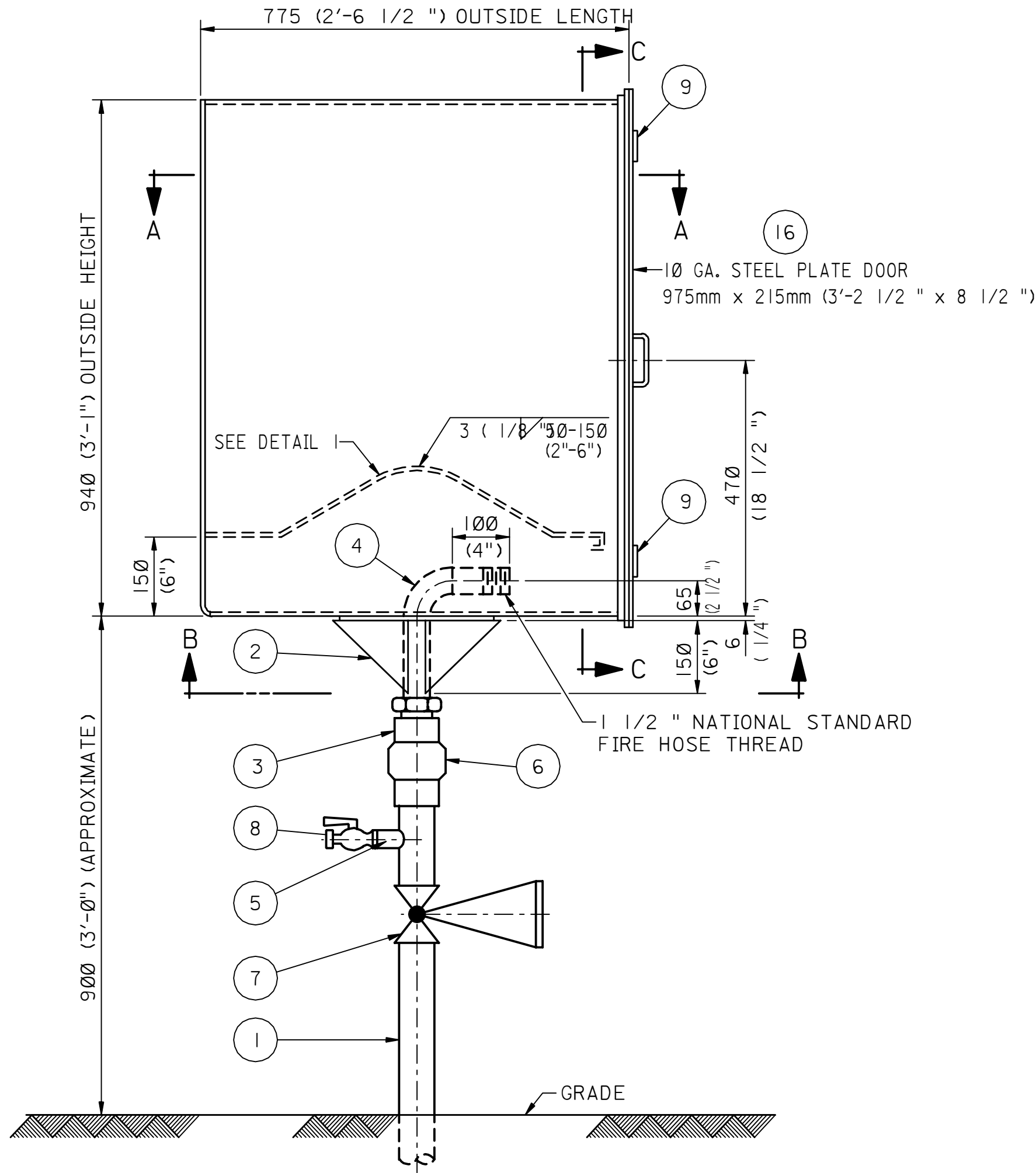
ELEVATION
