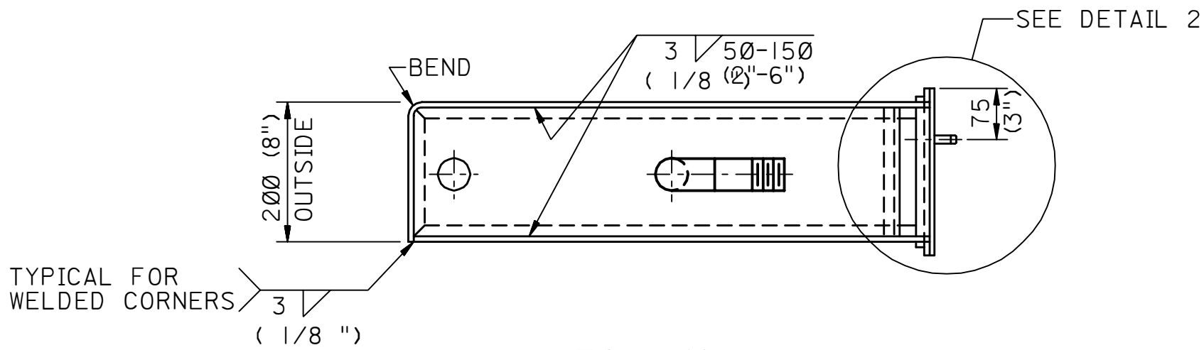
SECTION A-A
