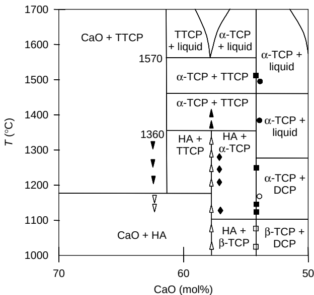
Figure 6.23 Part of the phase diagram of \text{CaO}-\text{P}_2\text{O}_5 under a water pressure of 500 mmHg (see text for identification of the various phases) (after Ribaud, 1973). Reproduced by permission of Lavoisier SAS from P.V. Ribaud, 'Composition et stabilité de phases à structure d'apatite dans le système \text{CaO}-\text{P}_2\text{O}_5 -oxyde de fer- \text{H}_2\text{O} à haute température', Ann. Chim. , 8, 1807–1813 (1973)
