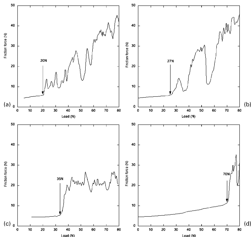
a DLC; b DLC/Ti; c DLC/TiN/Ti; d DLC/Ti/TiN/TiCN
