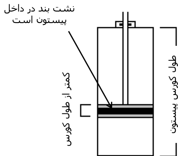
پمپ پیستونی
