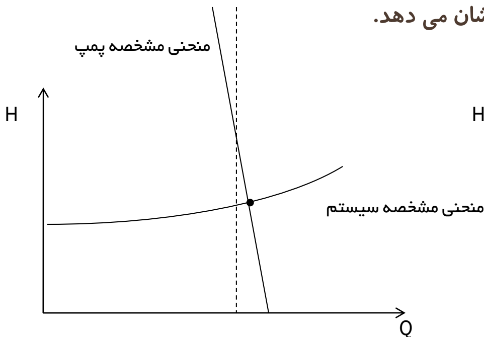
نقطه کار در پمپ های جابجایی
