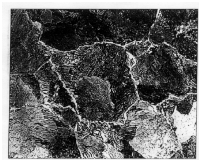
شکل 8 فولاد هایپروکتوید که ساختار آن شامل پرلیت و شبکه ای از سمنتیت (پرویوتکتوید) در مرز دانه های آستنیت اولیه است.
