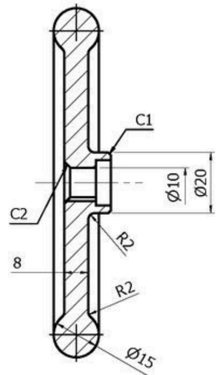
SECTION A-A
