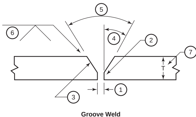
Groove Weld
