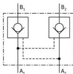
شکل (۲۴): نماد شیر یکطرفه دابل با عملکرد پیلوتی
