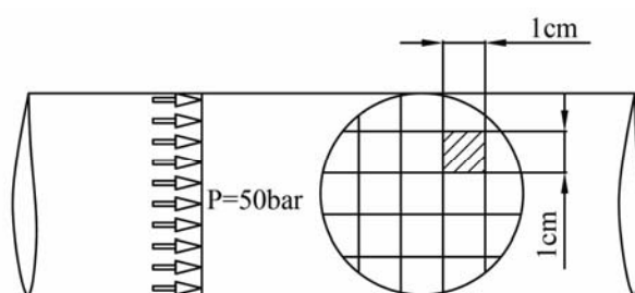
شکل (۴): نیروی ناشی از فشار روغن در لوله
