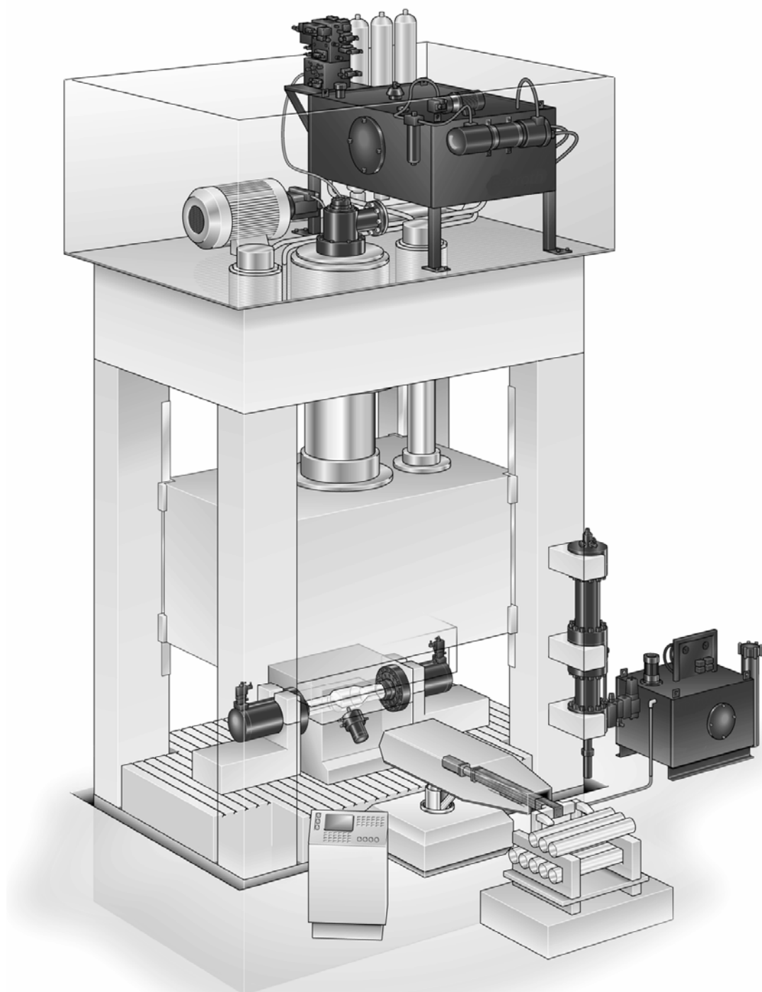
شکل (۲۷): پرس هیدرولیک به عنوان یک سیستم هیدرولیک نمونه
