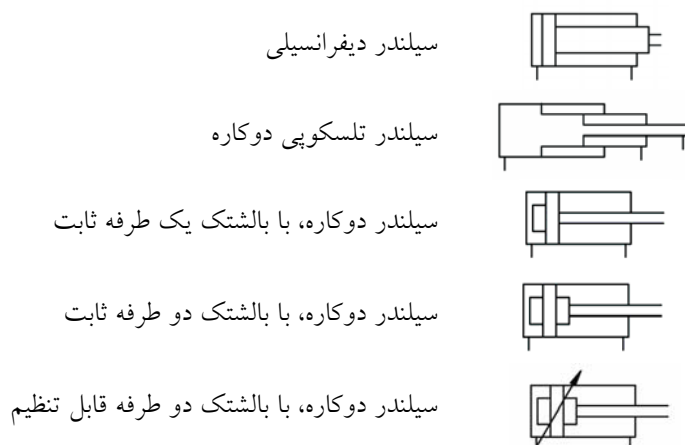
شکل (۲۱): نماد سیلندره‌ای دوطرفه
