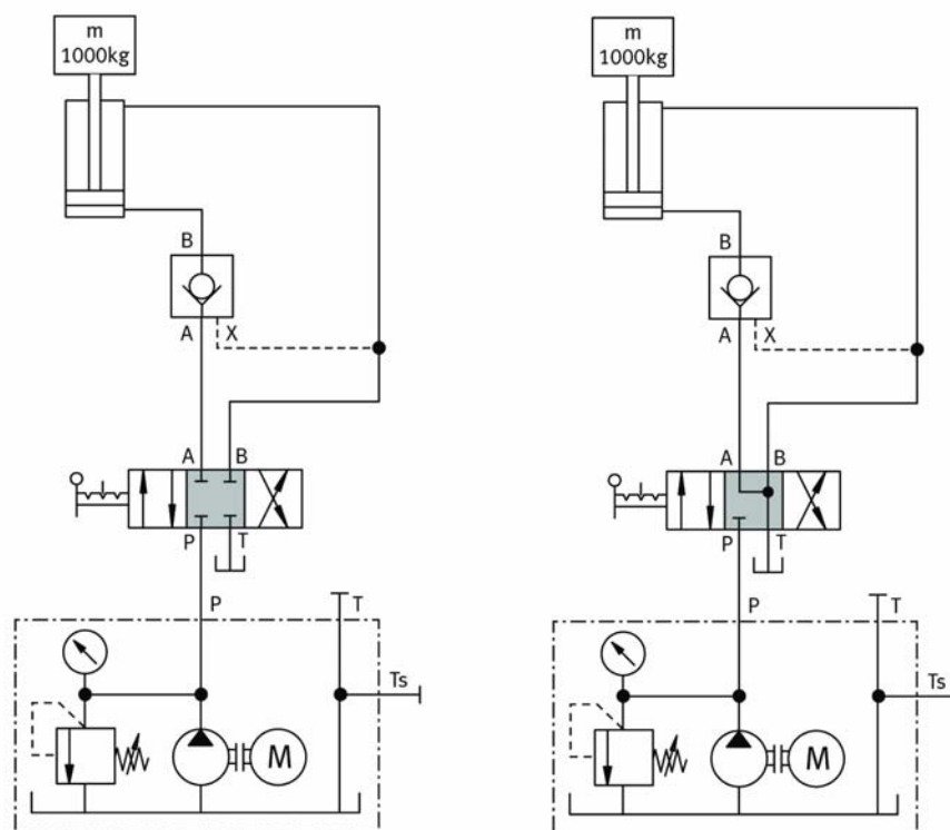
شکل (۶۱): تحریک شیر یکطرفه توسط شیر 4/3
