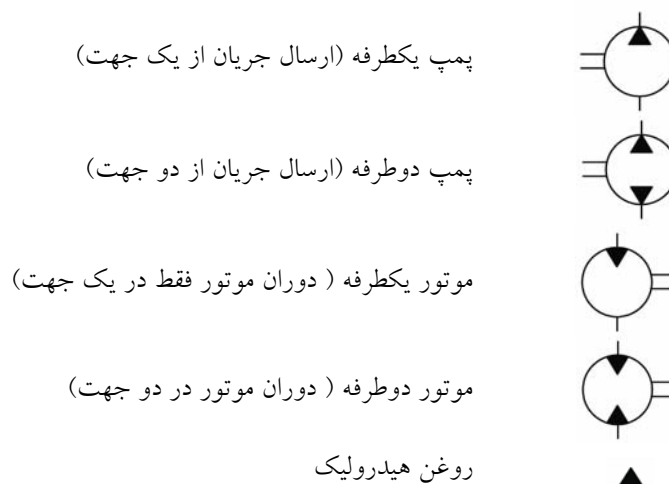
شکل (۸) : نماد پمپ و موتور با جابجائی ثابت
