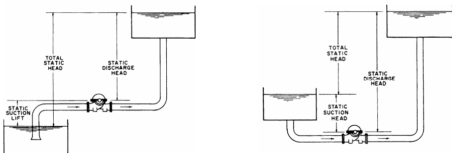
شکل (۱-۵): ارتفاع استاتیکی
