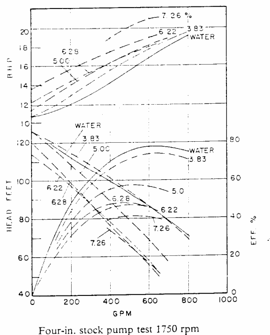
شکل (۶-۷): تأثیر ذرات جامد بر منحنی‌های مشخصه پمپهای گریزازمرکز
