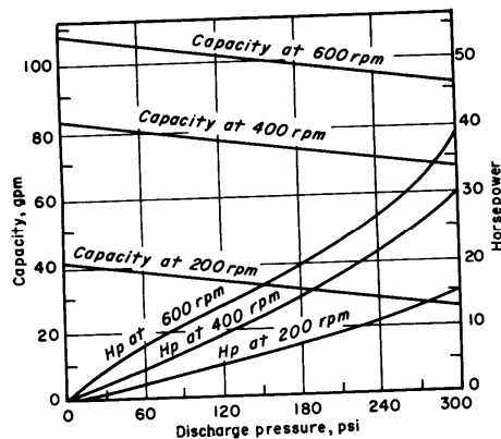
شکل (۱۸-۱): منحنی مشخصه یک پمپ دنده ای.
