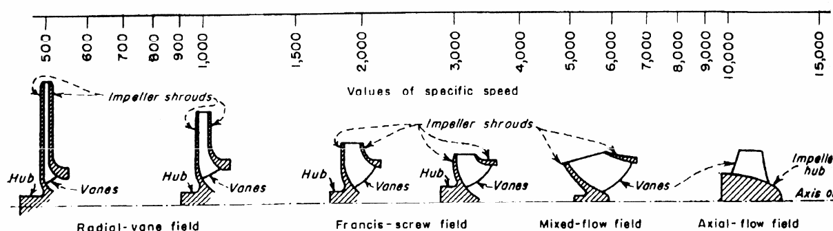
شکل (۴-۸): تغییرات سرعت مخصوص با شکل پروانه
