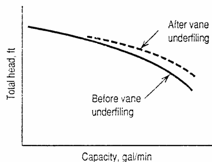
شکل (۸-۲): تأثیر تیز کردن لبه زیرین تیغه‌ها بر روی منحنی مشخصه پمپ
