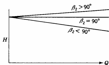
شکل (۱-۲): منحنی مشخصه پمپهای گریز از مرکز
