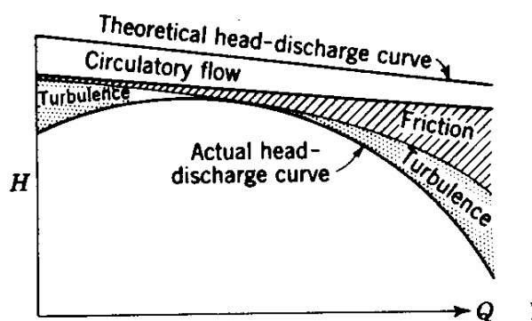
شکل (۲-۴): از دست رفت ارتفاع در پمپهای گریز از مرکز
