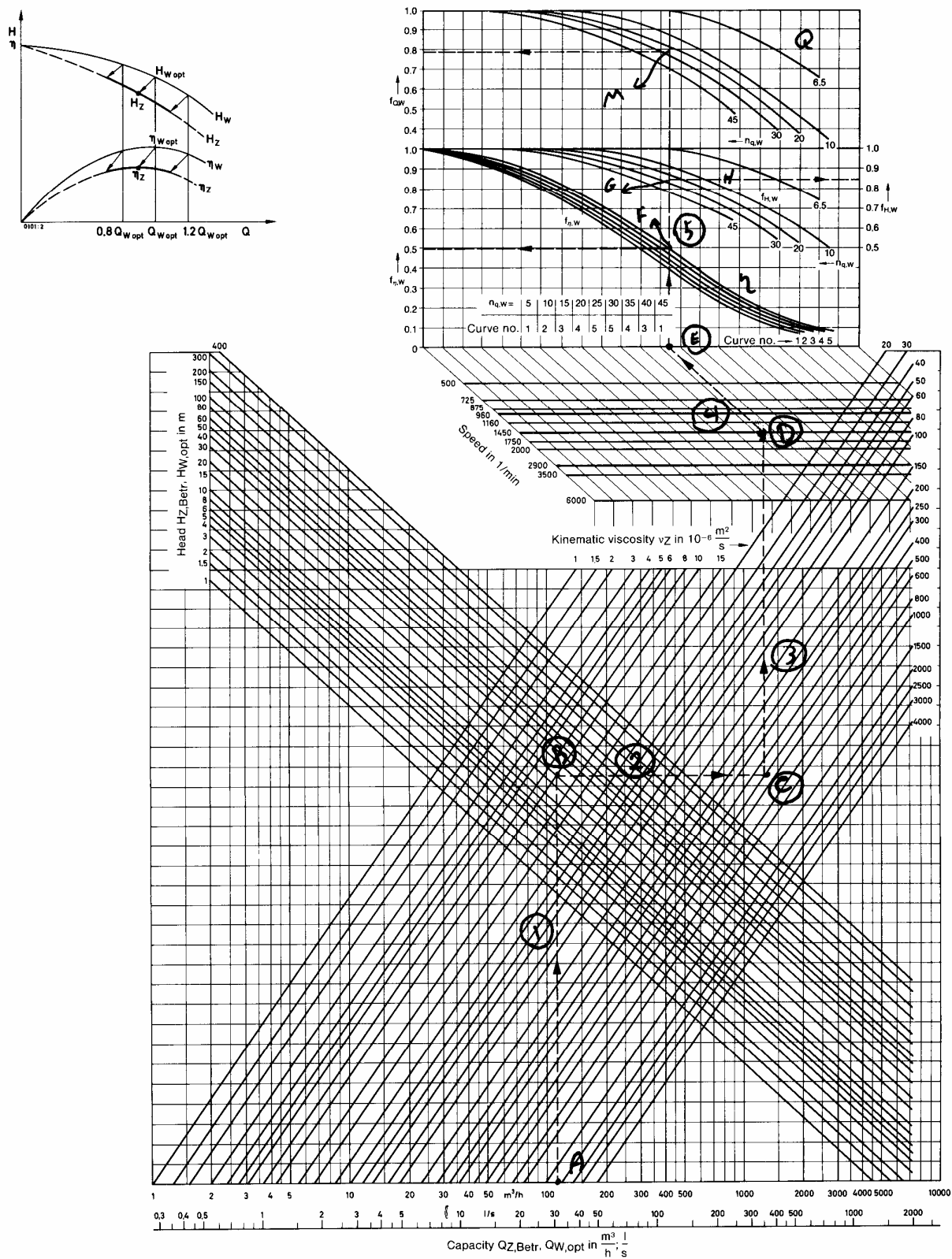
شکل (۳-۶): تعیین ضرایب اصلاح مشخصه‌های پمپ برای مایعات غیر از آب
