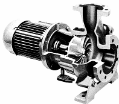
شکل (۱-۳): پمپ پیچکی یک طبقه با یک مکش در قسمت ته آن و پروانه نیمه بسته
