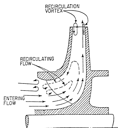
شکل (۲-۶): جریان گردشی در مکش پمپ
