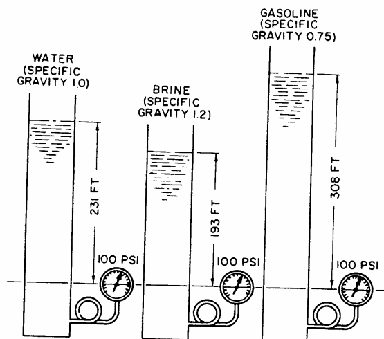
شکل (۱-۴): تأثیر وزن مخصوص بر روی ارتفاع استاتیکی جهت دستیابی به فشار معین.
