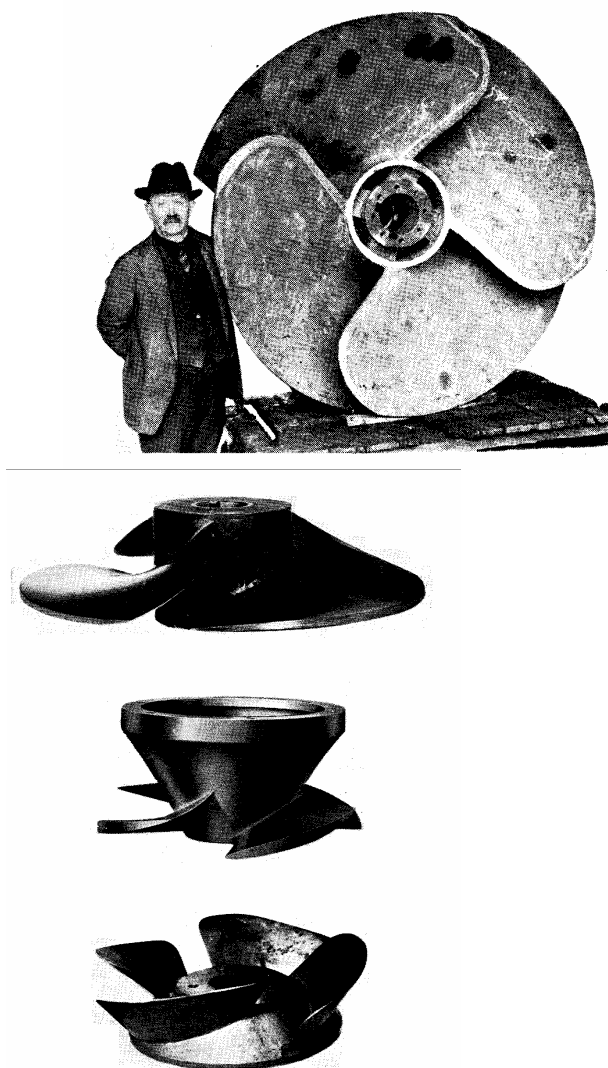
شکل (۱۲-۳): انواع پروانه‌های مورد استفاده در پمپهای ملخی
