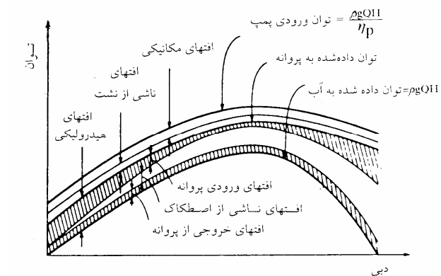
شکل (۹-۲): ازدست رفت انرژی در پمپ
