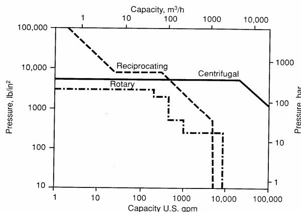
شکل (۱-۳): محدوده به کارگیری انواع پمپها.
