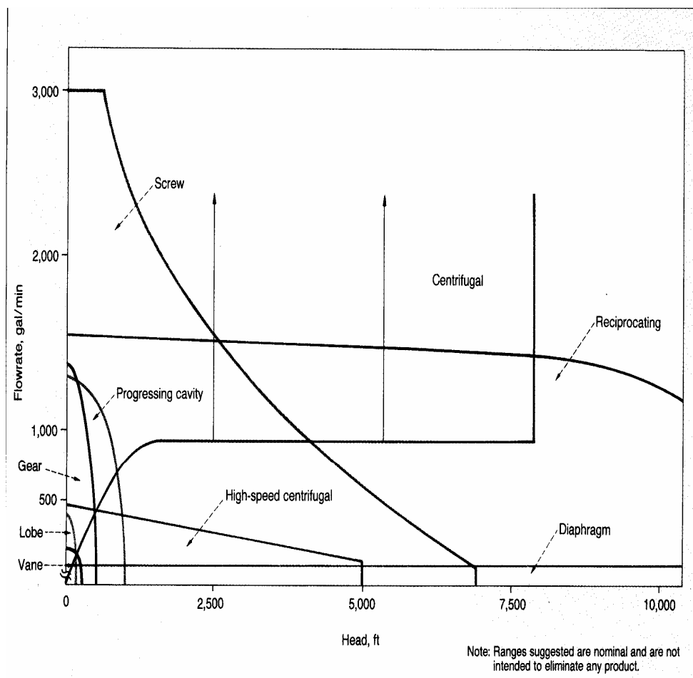
شکل (۱-۱۶): دامنه کاربرد انواع پمپها
