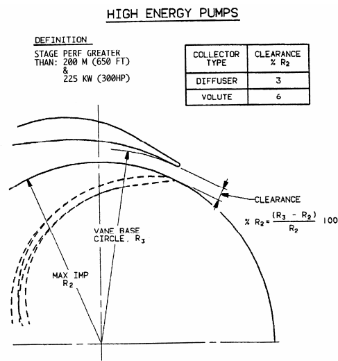
شکل (۴-۱۵): لقی محوری بین پروانه و تیغه های ثابت (فاصله هوایی B)
