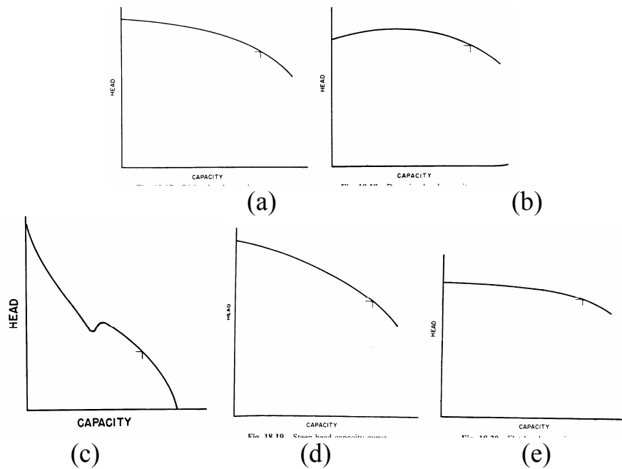
شکل (۱۰-۱۲): انواع منحنی‌های مشخصه پمپهای گریز از مرکز
