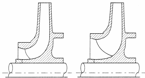
شکل (۷-۱۳): تغییر چشمه پروانه جهت کاهش NPSHR
