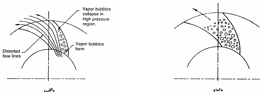
شکل (۷-۶): کاویتاسیون جزئی (الف) و کلی (ب)
