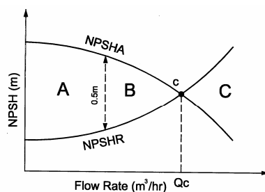
شکل (۷-۱۰): منحنی تغییرات NPSHA و NPSHR بر حسب دبی
