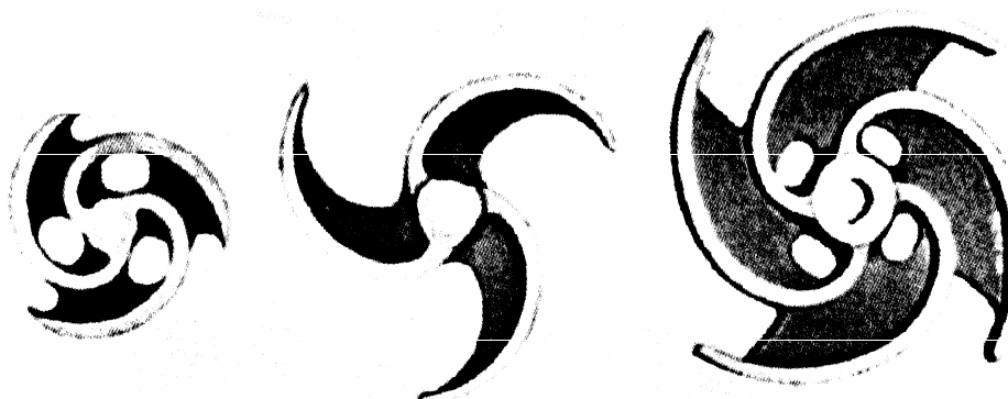
شکل (۴-۹): پروانه های باز - شکلهای چپ و راست با صفحات نگهدارنده تقویت شده اند.
