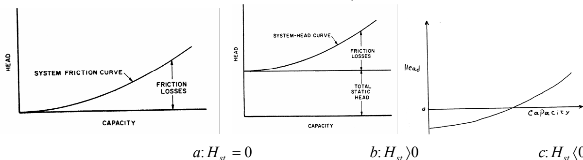
شکل (۱-۶): منحنی مشخصه سیستم در انواع سیستم‌های انتقال مایعات.
