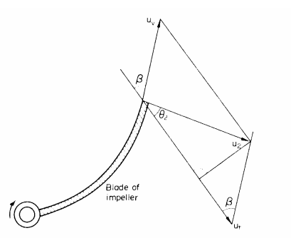
شکل (۱-۱): مثلث سرعت در لبه یک تیغه پروانه
