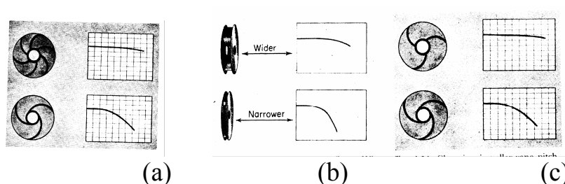
شکل (۷-۲): تأثیر ویژگی‌های پروانه بر روی منحنی مشخصه پمپ
