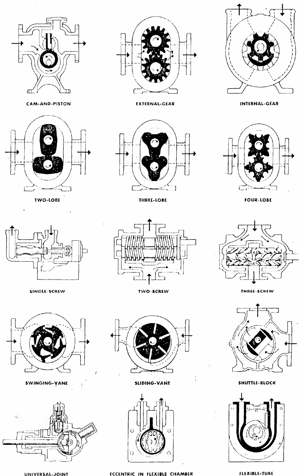
شکل (۱۷-۱): انواع پمپهای دورانی.
