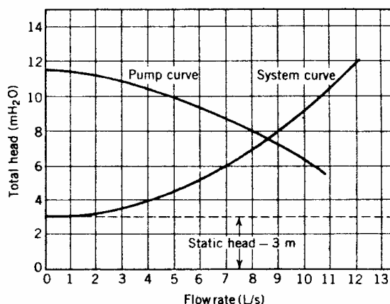
شکل (۸-۱): نقطه کار در سیستم های پمپاژ.
