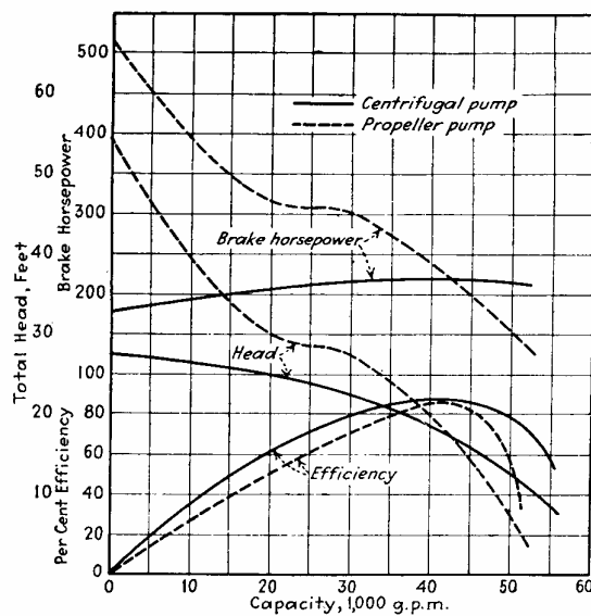
شکل (۱۳-۳): مقایسه منحنی مشخصه پمپهای ملخی و پیچکی
