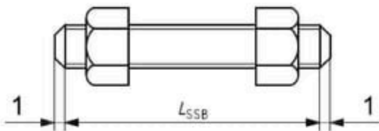
c) Stud bolt with nuts
